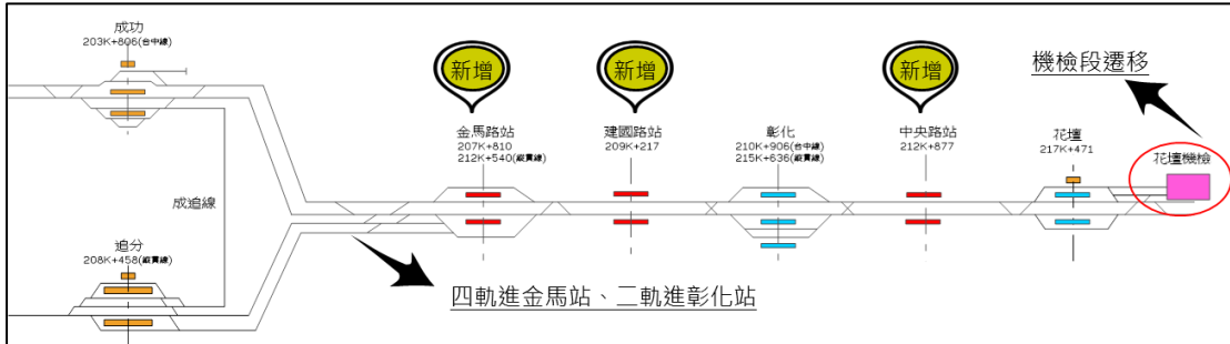
圖 5：彰化市鐵路高架化計畫增站示意圖
