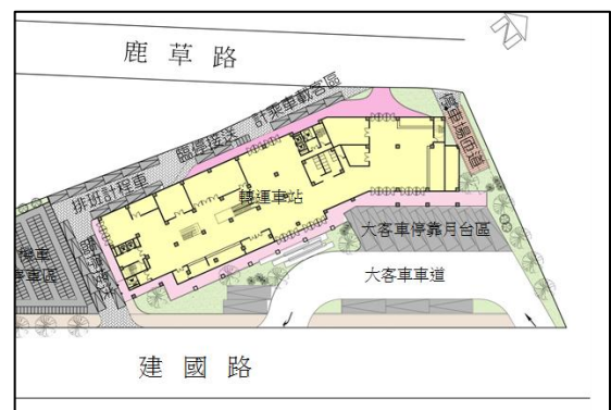
圖10：鹿港轉運站平面配置示意圖
