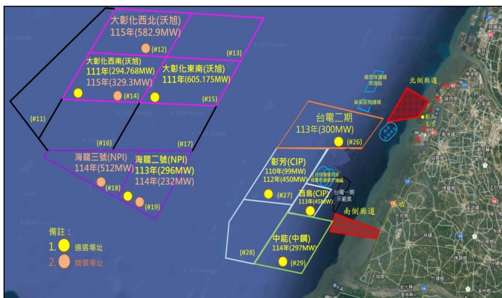
圖 9：離岸風電分布圖
