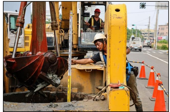
圖 21：和美鎮污水主次幹管及分支管網施工情形
