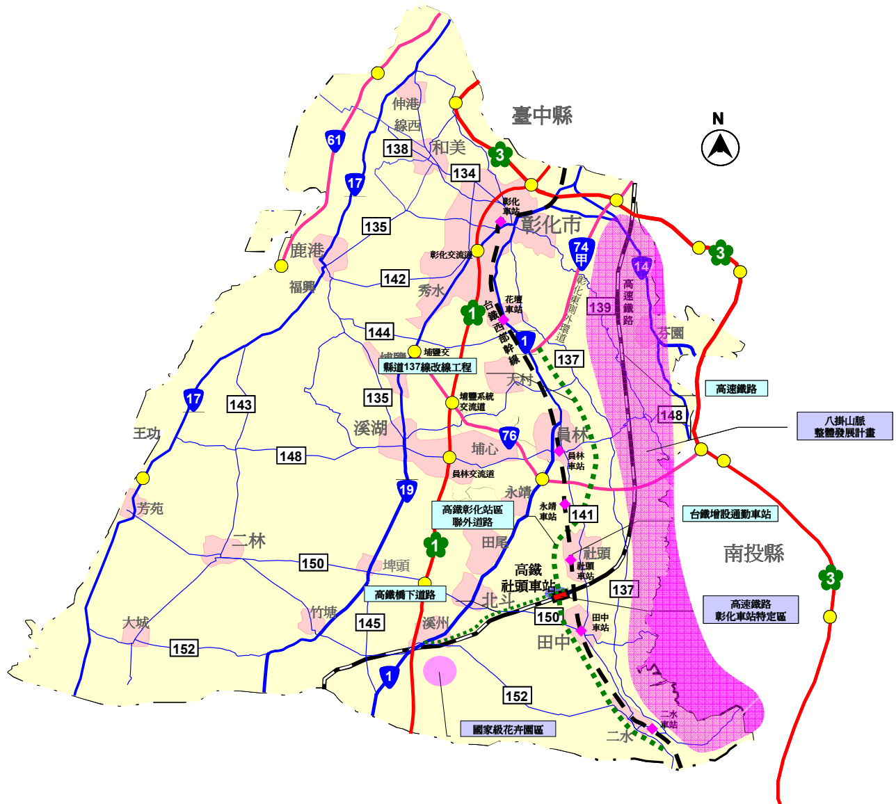
圖 2.7-1 相關建設計畫分佈區位示意圖
